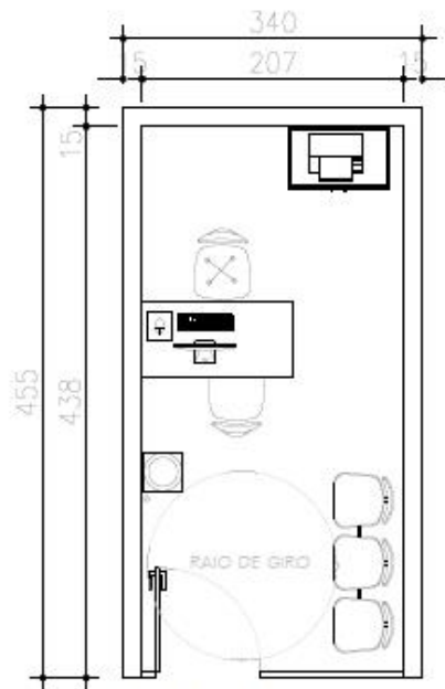
Balcão Expresso Proposta 1 Guichê de Atendimento
